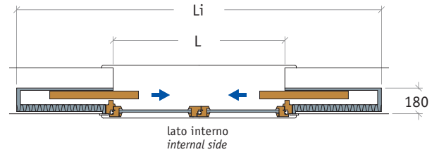
Controtelaio doppio Single Frame, double
