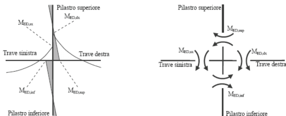
Figura C4.1.2 - Diagramma delle sollecitazioni e schema dei momenti trasmessi al nodo con momenti d'estremità discorde
