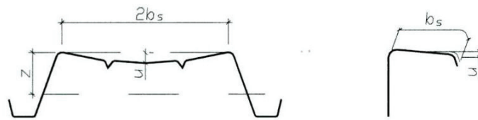
Figura C4.2.25 -Incurvamento delle piattabande
