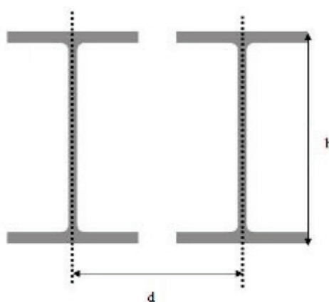
Figura C3.3.28 – Travi parallele
