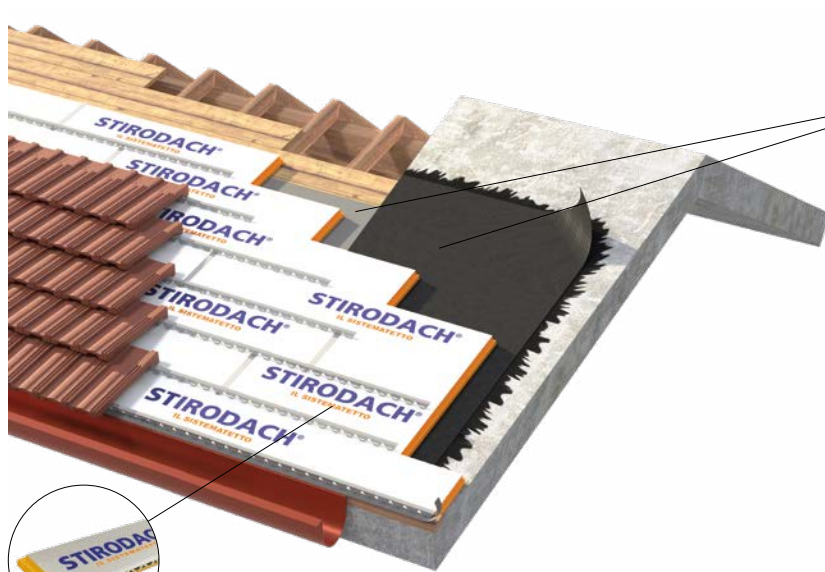
ELEMENTO TERMOISOLANTE STIRODACH - pag. 39
